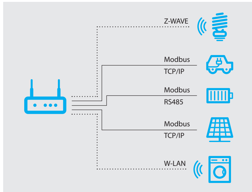
Abbildung 5: Beispielhafter HEMS-Aufbau mit unterschiedlichen Kommunikationskanälen
